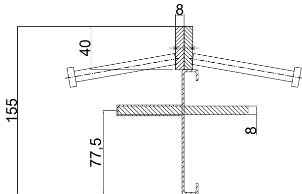
CONECTO DOWEL 08NA40-5D-T8 h=155 Section Scale 2:1
