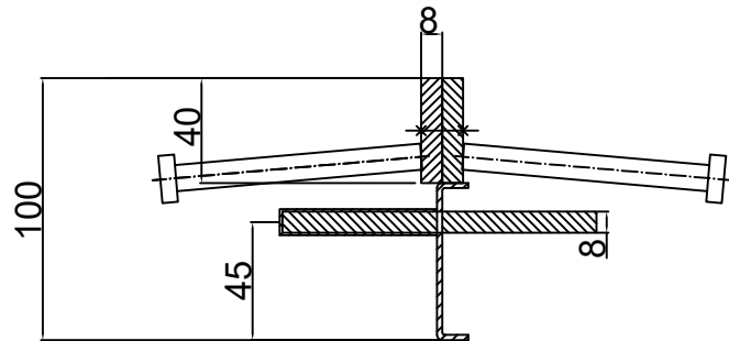
CONECTO DOWEL 08NA40-5D-T8 h=100 Section Scale 2:1
