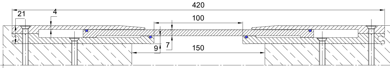
Conecto AL 420/21 Section SCALE 1:1,75
